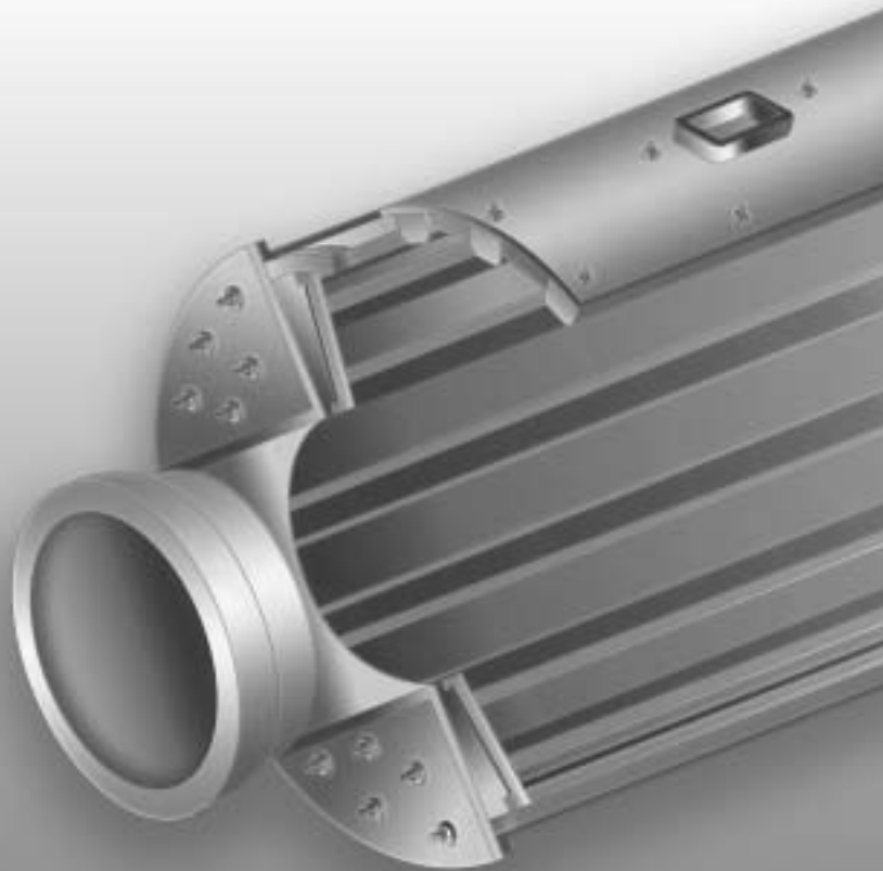
Корпусная пластина
